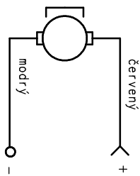
SCHEMA ZAPOJENÍ
